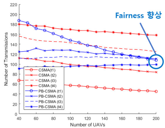
그림 3. CSMA와 PB-CSMA 구역별 전송 횟수
