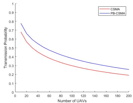
그림 2. CSMA와 PB-CSMA 전송 성공률
