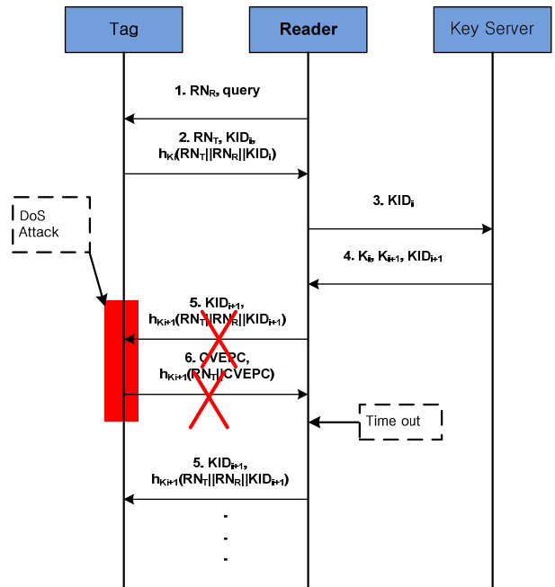
그림 2. 제안하는 인증 프로토콜에서의 DoS 공격에 대처하는 과정
